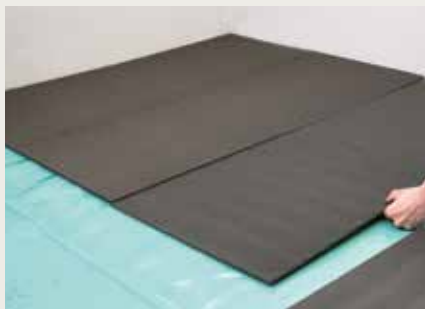
QUICKHEAT-ISOLATIEPLATEN Isolatieplaten. 120 × 50 × 0,7 cm. 10 platen/verpakking. 0,6 m 2 /plaat, 6 m 2 /verpakking. Dikte: 7 mm. Het gebruik van een damp scherm is aanbevolen. Plaats PE-folie PGUSCRSCREEN34 onder QuickHeat-isolatieplaten en ook op QuickHeat-folies.
